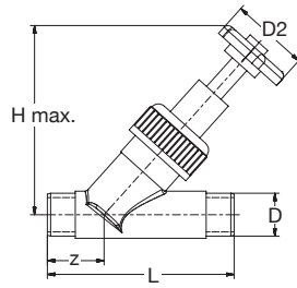
BR PVC-U Ventil Schrägsitz Runddichtring-EPDM grau BR PVC-U Valve angle seat O-Ring-gasket-EPDM grey
