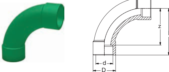
BR PP-RCT Bogen 90° grün
