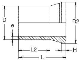
BR PP-INDUSTRIAL Verschraubung Einlegeteil lang st SDR11 grau BR PP-INDUSTRIAL Union Insert-part long butt SDR11 grey
