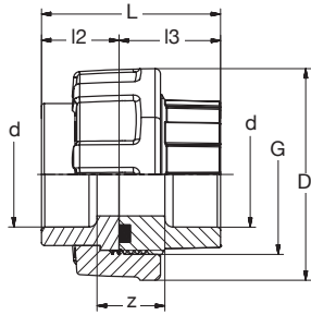
BR PP-RCT Verschraubung Runddichtung-EPDM 20°C/1,0MPa grün BR PP-RCT Union O-Ring-gasket-EPDM 20°C/1.0MPa green
