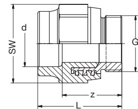
BR PP-RCT-RG/LFB Verschraubung Schraubteil flachdichtend grün BR PP-RCT-Bronze/LFB Union Srew-part flat-sealing green
