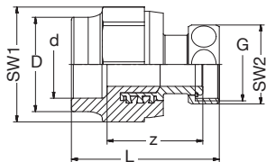
BR PP-RCT-RG/LFB A-Verschraubung IG-zyl für Armaturen + Wasserzähler mit Flachdichtung-EPDM grün
